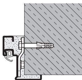
rohová zárubeň do pohledového zdiva/betonu nutno uvést v objednávce
