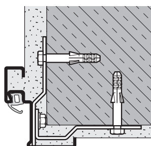
rohová zárubeň standard
