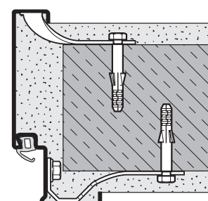
U-zárubeň do zdiva/betonu
