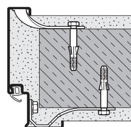
U-zárubeň do zdiva/betonu
