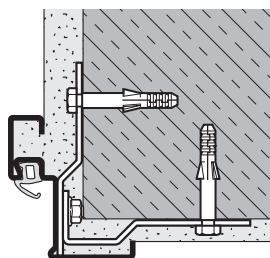
rohová zárubeň standard
